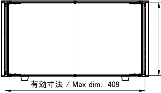
C-C ( 1 : 6.5 )
