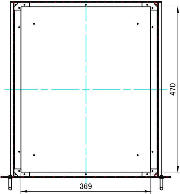
B-B ( 1 : 6.5 )
