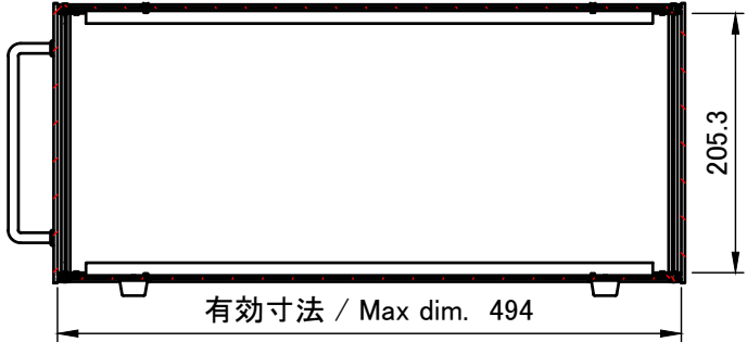
A-A ( 1 : 6.5 )
