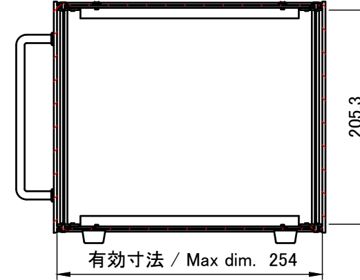
A-A (1:5)
