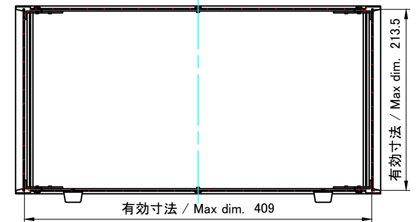
C-C ( 1 : 4.5 )
