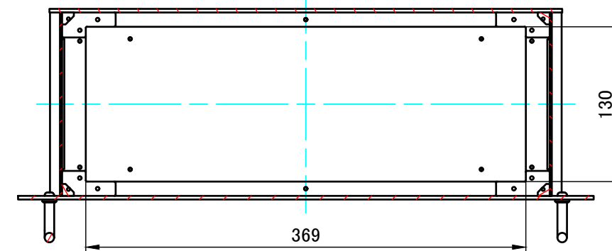
B-B ( 1 : 4.5 )
