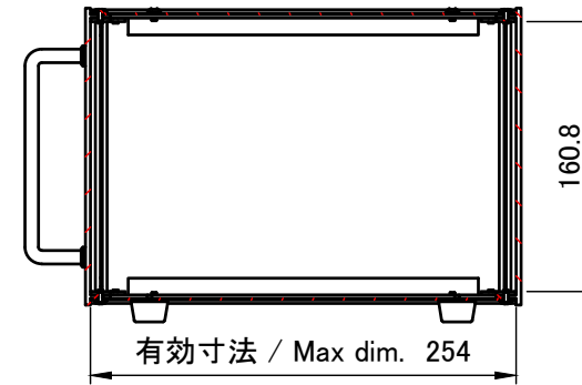
A-A (1:5)
