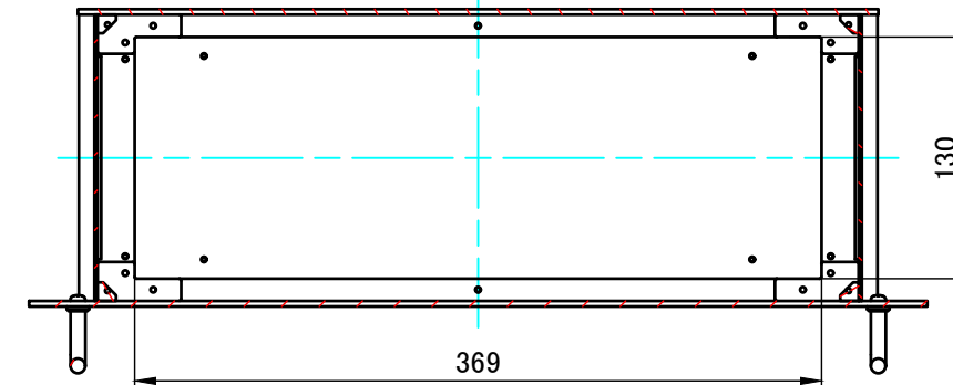
B-B ( 1 : 4.5 )
