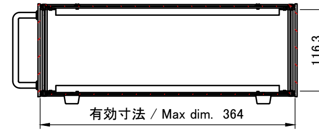
A-A ( 1 : 5.5 )
