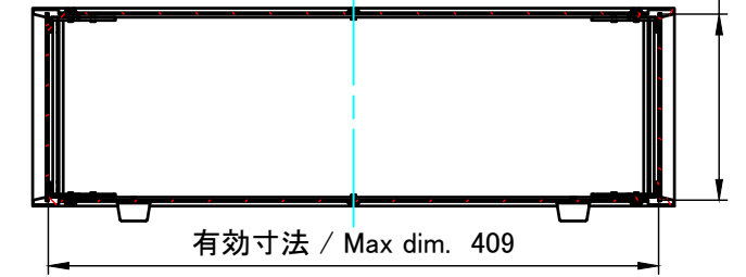
C-C ( 1 : 5.5 )
