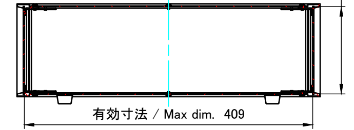
C-C ( 1 : 5.5 )
