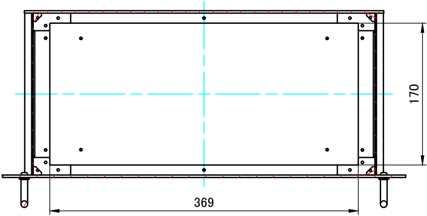
B-B ( 1 : 4.5 )
