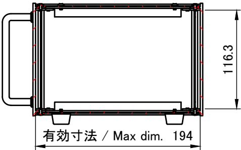
A-A ( 1 : 4.5 )
