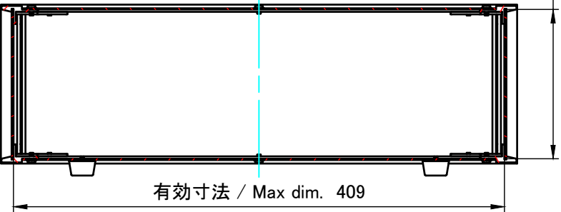
C-C ( 1 : 4.5 )
