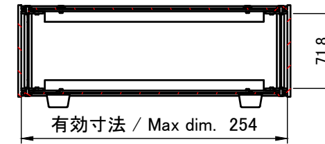
A-A (1:5)
