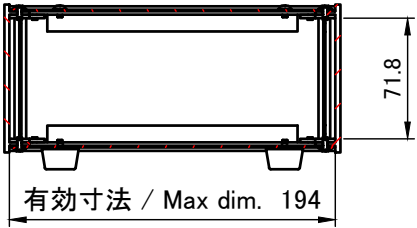
A-A ( 1 : 4.5 )
