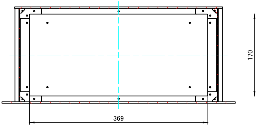
B-B ( 1 : 4.5 )
