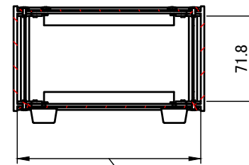
A-A ( 1 : 4.5 )
