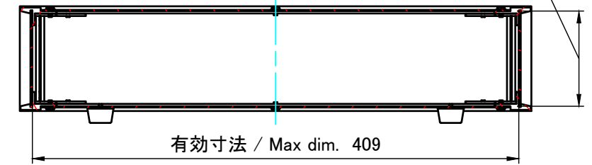
C-C ( 1 : 4.5 )
