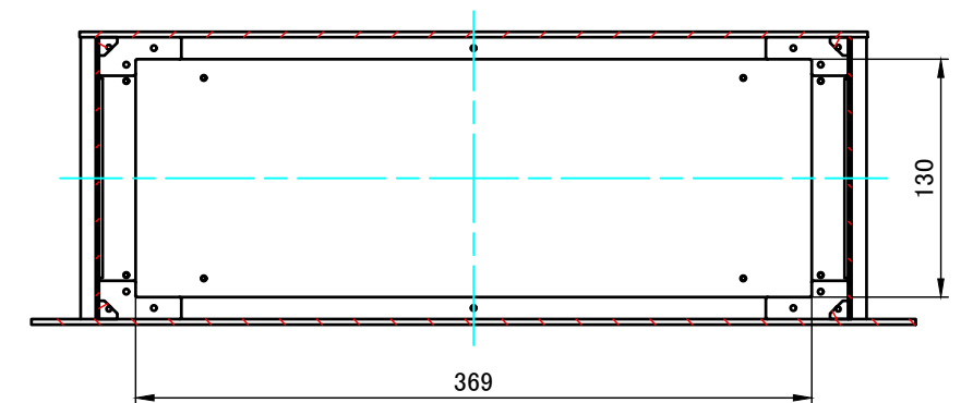
B-B ( 1 : 4.5 )
