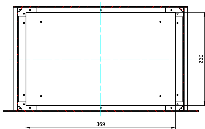
B-B ( 1 : 4.5 )
