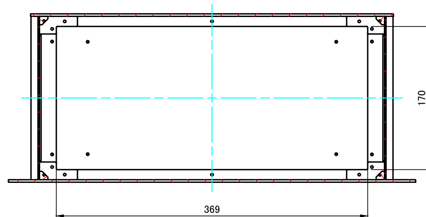
B-B ( 1 : 4.5 )
