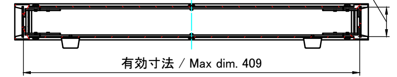
C-C ( 1 : 4.5 ) 有効寸法 / Max dim. 36
