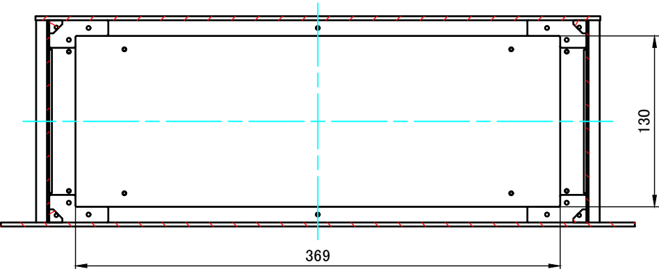
B-B ( 1 : 4 )
