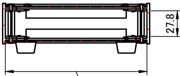
A-A ( 1 : 4 )
