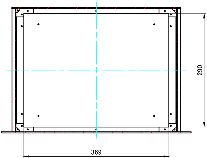
B-B ( 1 : 5.5 )
