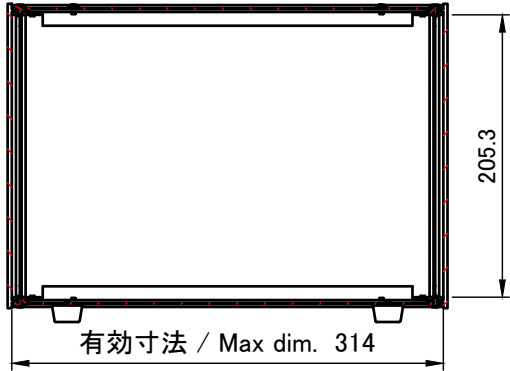
A-A ( 1 : 5.5 )
