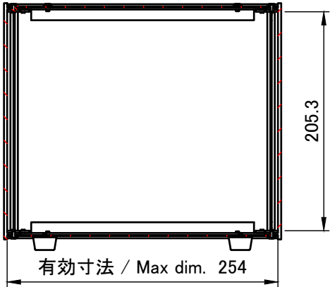
A-A ( 1 : 5 )
