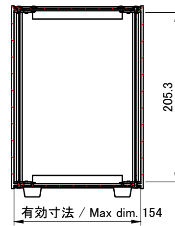
A-A ( 1 : 4.5 )
