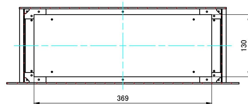
B-B ( 1 : 4.5 )
