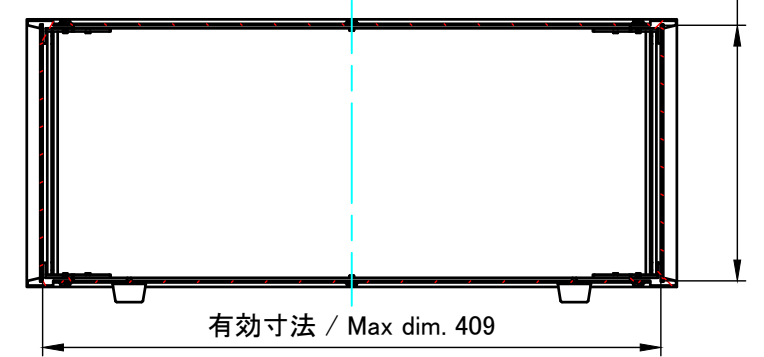
C-C ( 1 : 5 )
