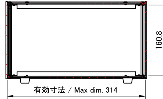
A-A ( 1 : 5 )
