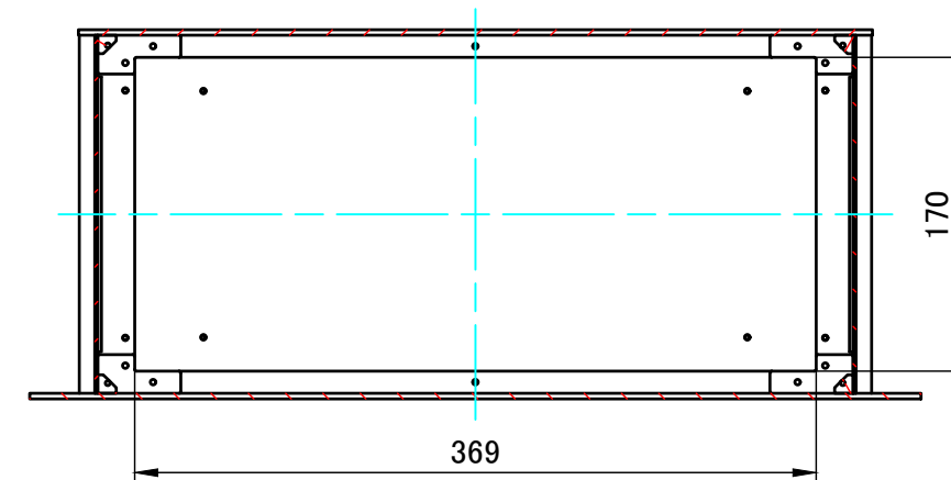
B-B ( 1 : 4.5 )
