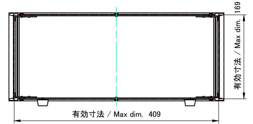
C-C ( 1 : 4.5 )
