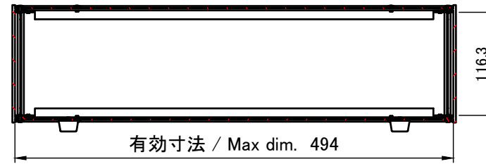
A-A (1:6)
