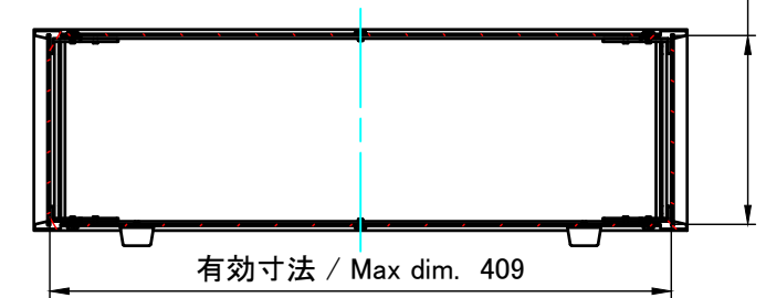
C-C ( 1 : 5.5 )
