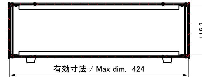
A-A ( 1 : 5.5 )
