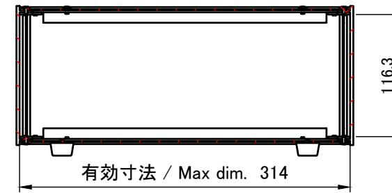
A-A (1:5)
