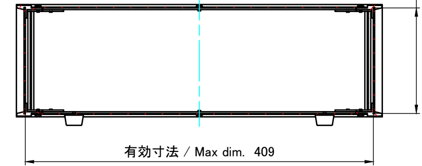
C-C ( 1 : 4.5 )
