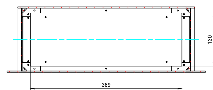
B-B ( 1 : 4.5 )
