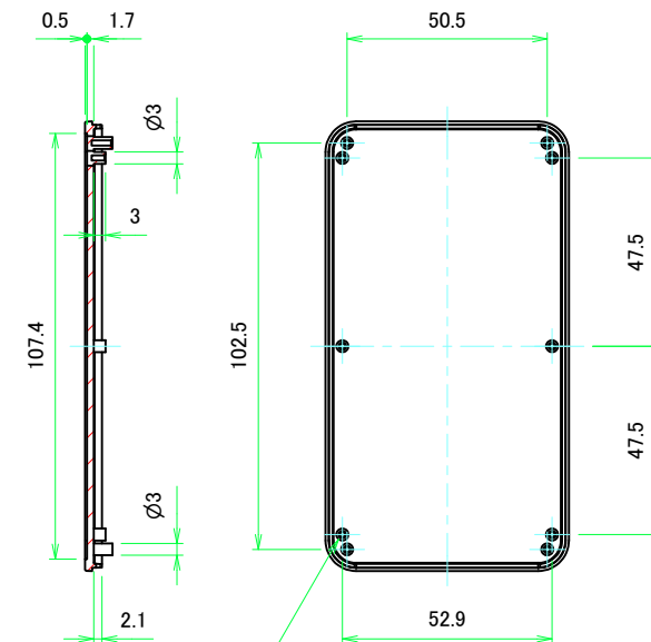
6-M1.6用基板取付ボス 6-M1.6 Boss
