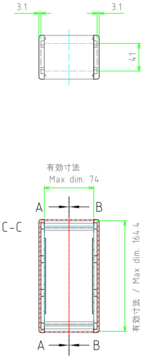
ハメ込みパネル(内視) Slide panel (Internal View)
