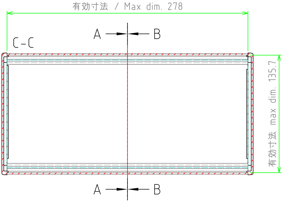
ハメ込みパネル(内視) / Slide panel (Internal View)
