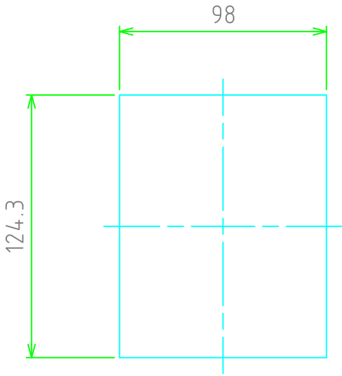
パネル表面 / Panel Frontside
