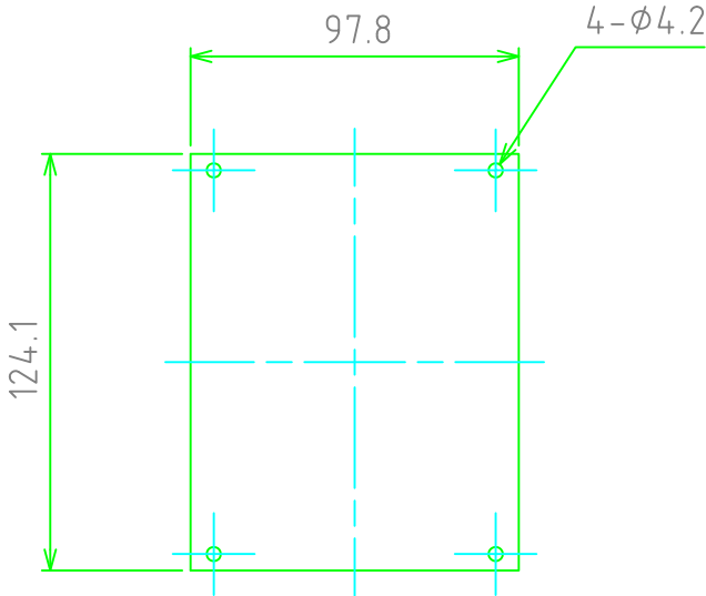
パネル表面 / Panel Frontside
