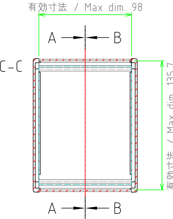
ハメ込みパネル(内視) Slide panel (Internal View)
