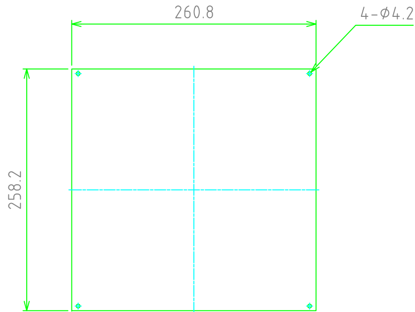
パネル表面 / Panel Frontside
