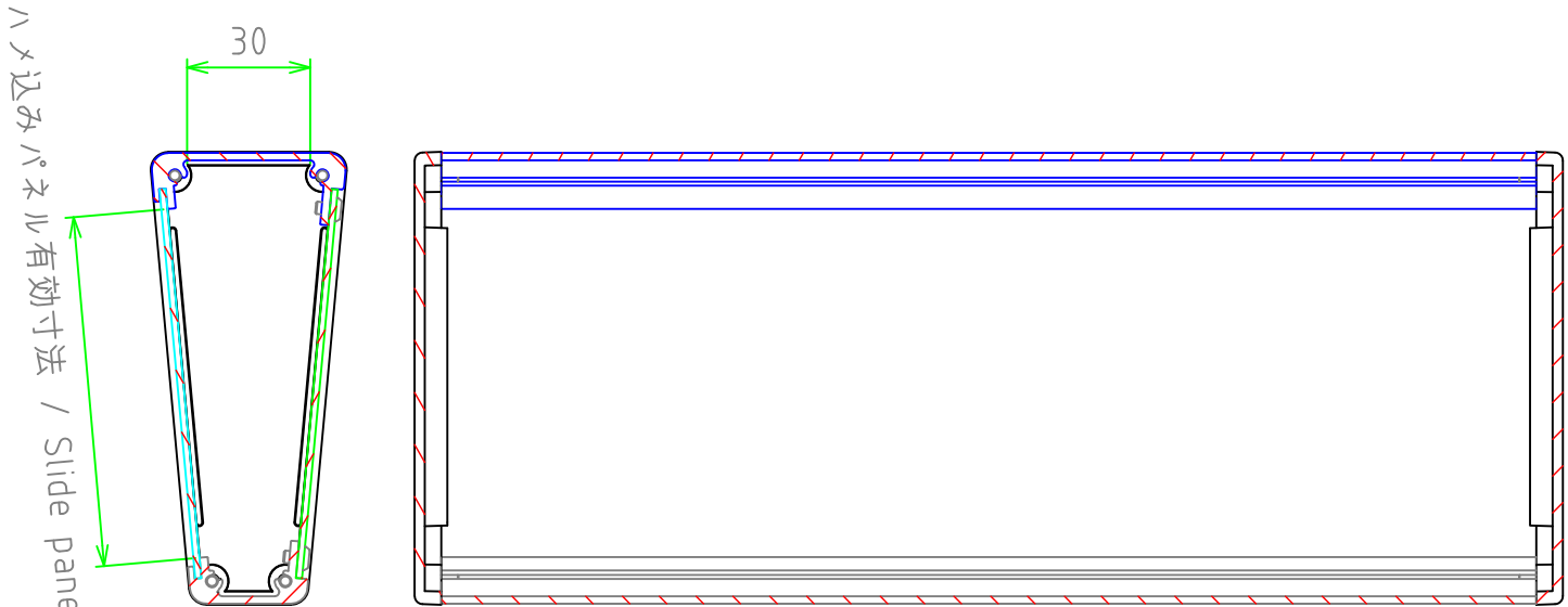
ハメ込みパネル(内視) Slide panel (Internal View)
