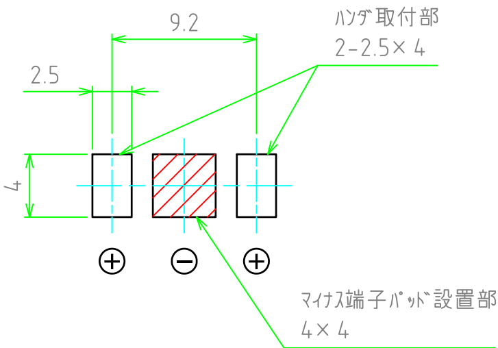
基板実装図
