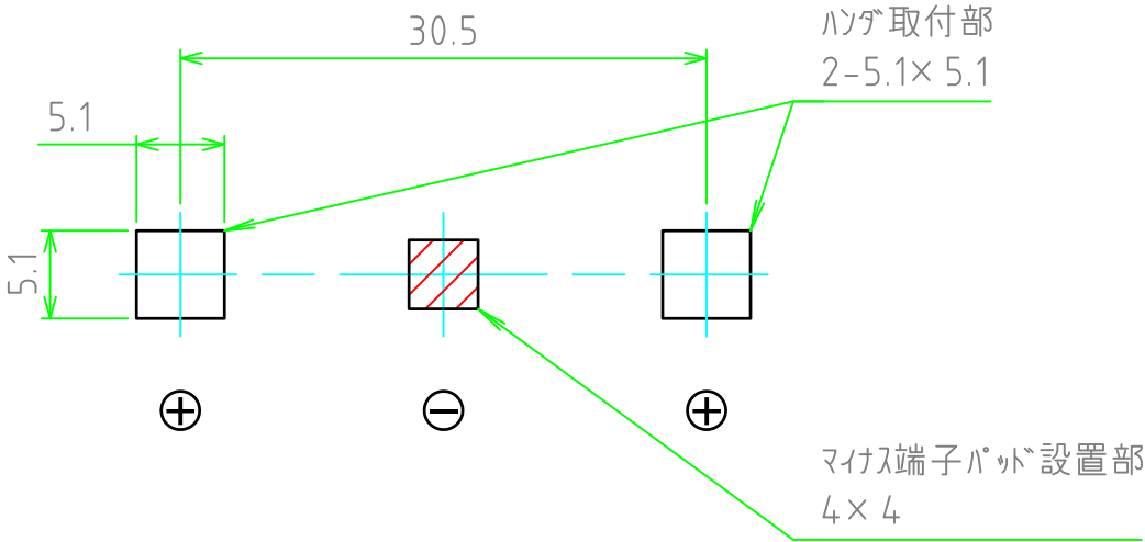
基板実装図
