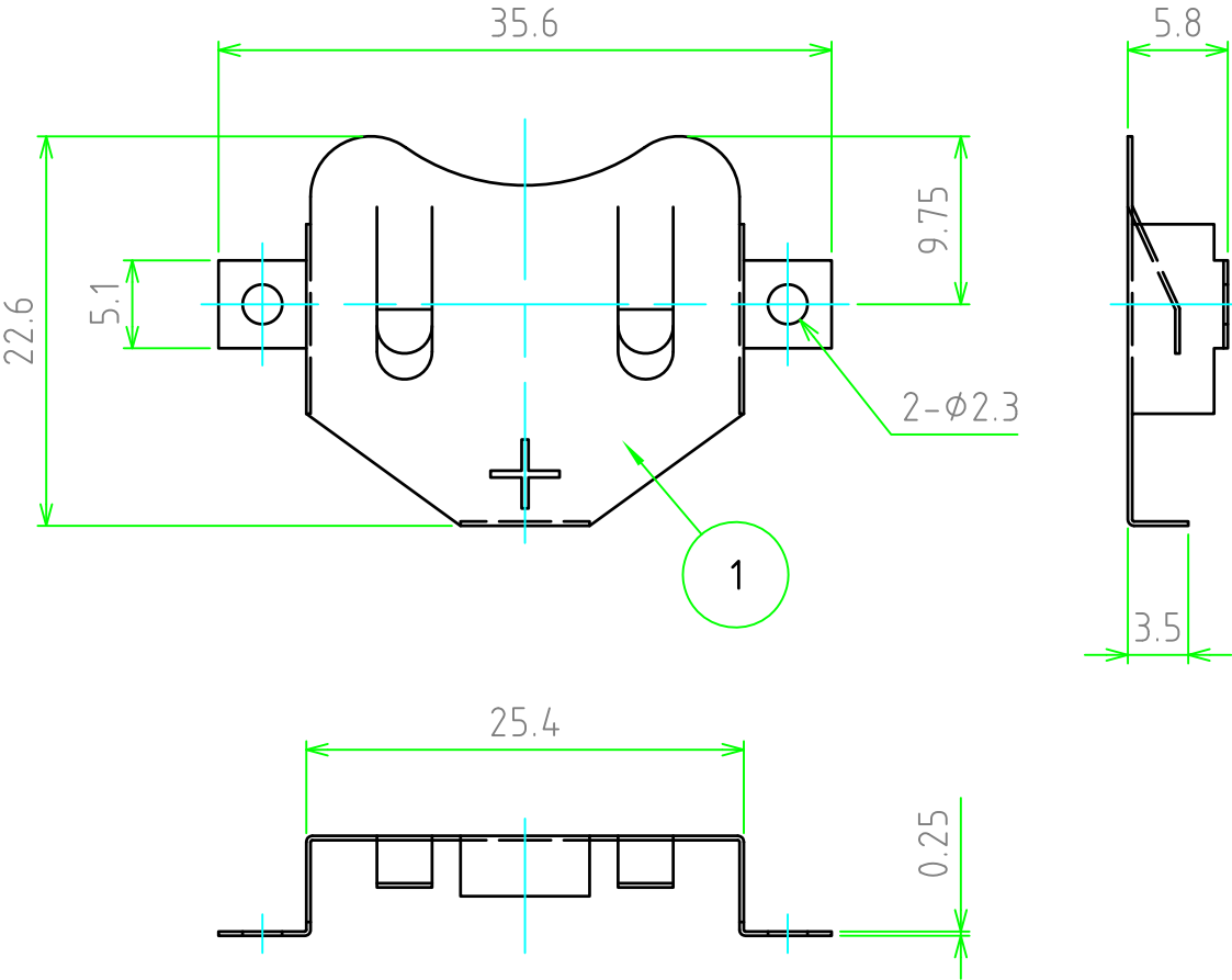
基板実装図
