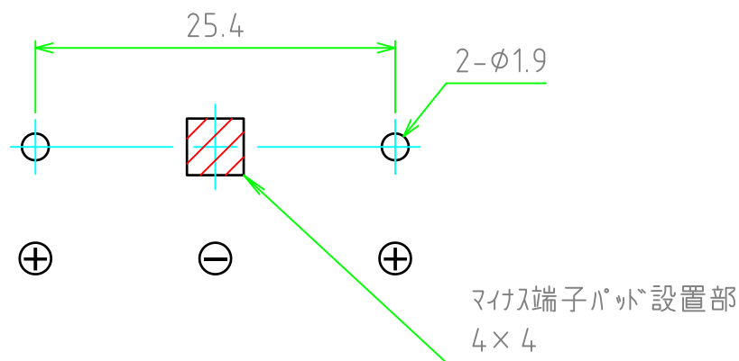
基板実装図
