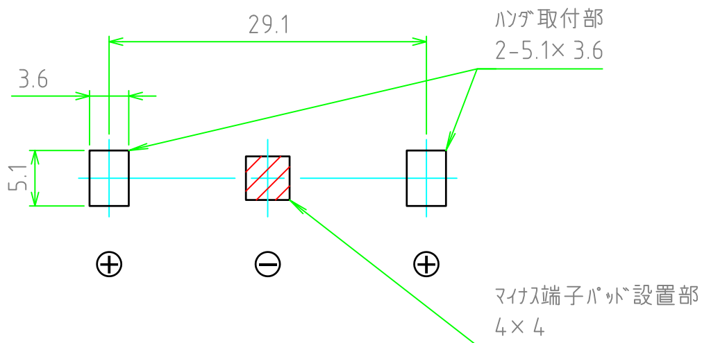
基板実装図
