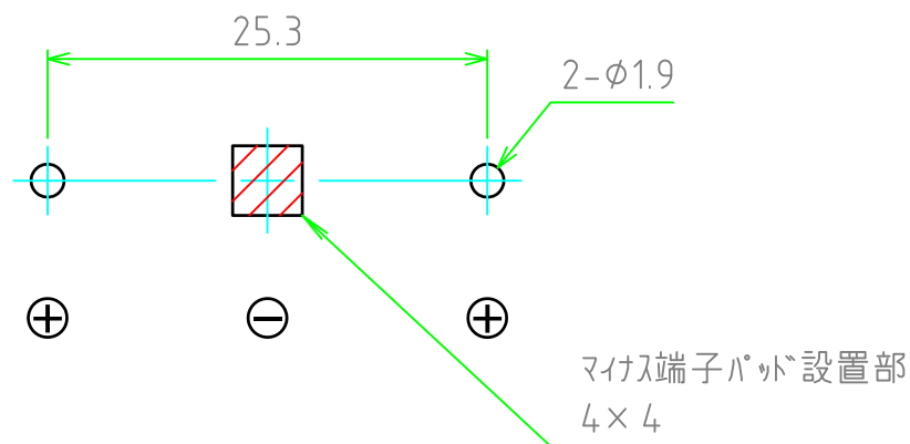
基板実装図
