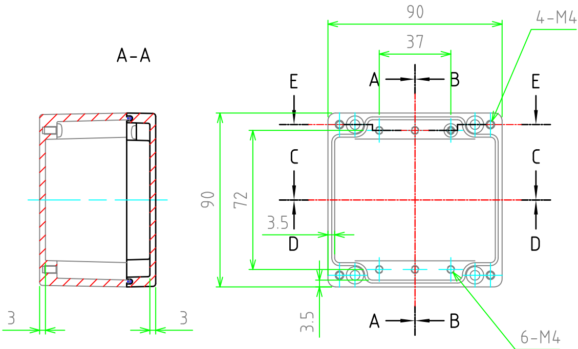
ボディー（内視） Base (Internal View)
