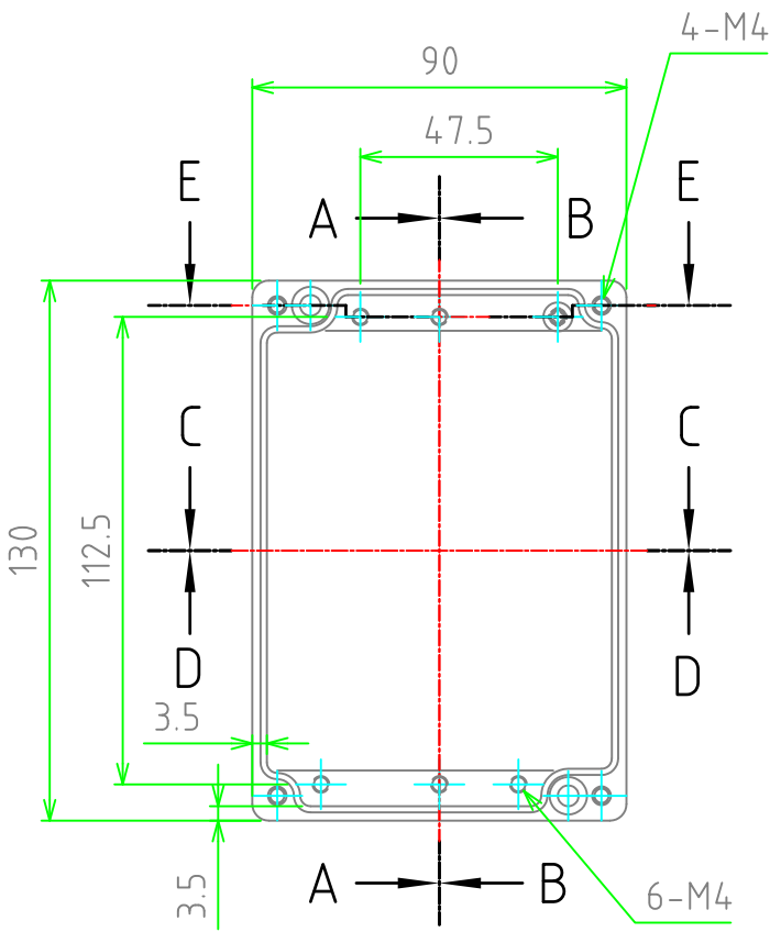
ボディー（内視） Base (Internal View)
