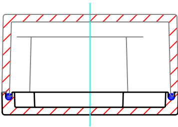
ボディー（内視） Base (Internal View)
