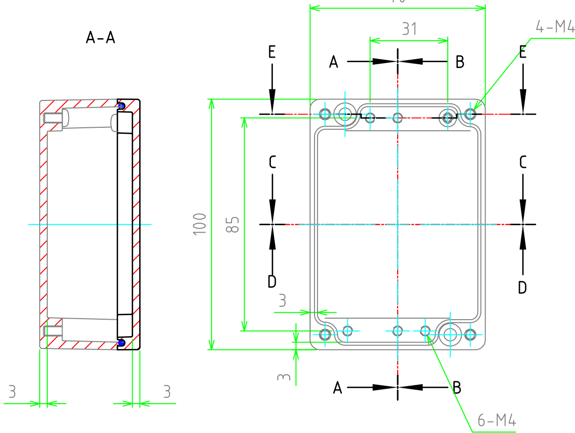
ボディー（内視） Base (Internal View)
