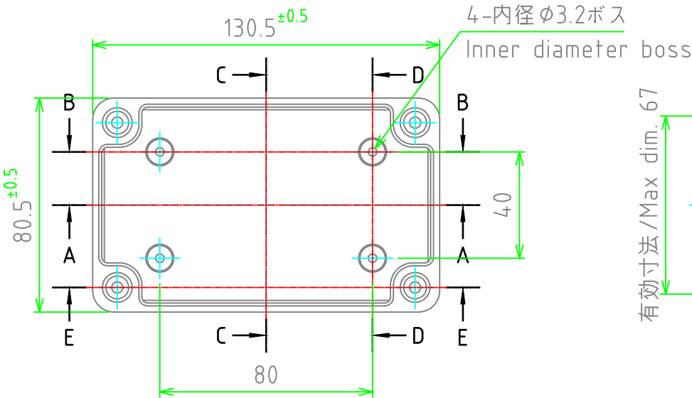
ボディー (内視) Body (Internal View)
