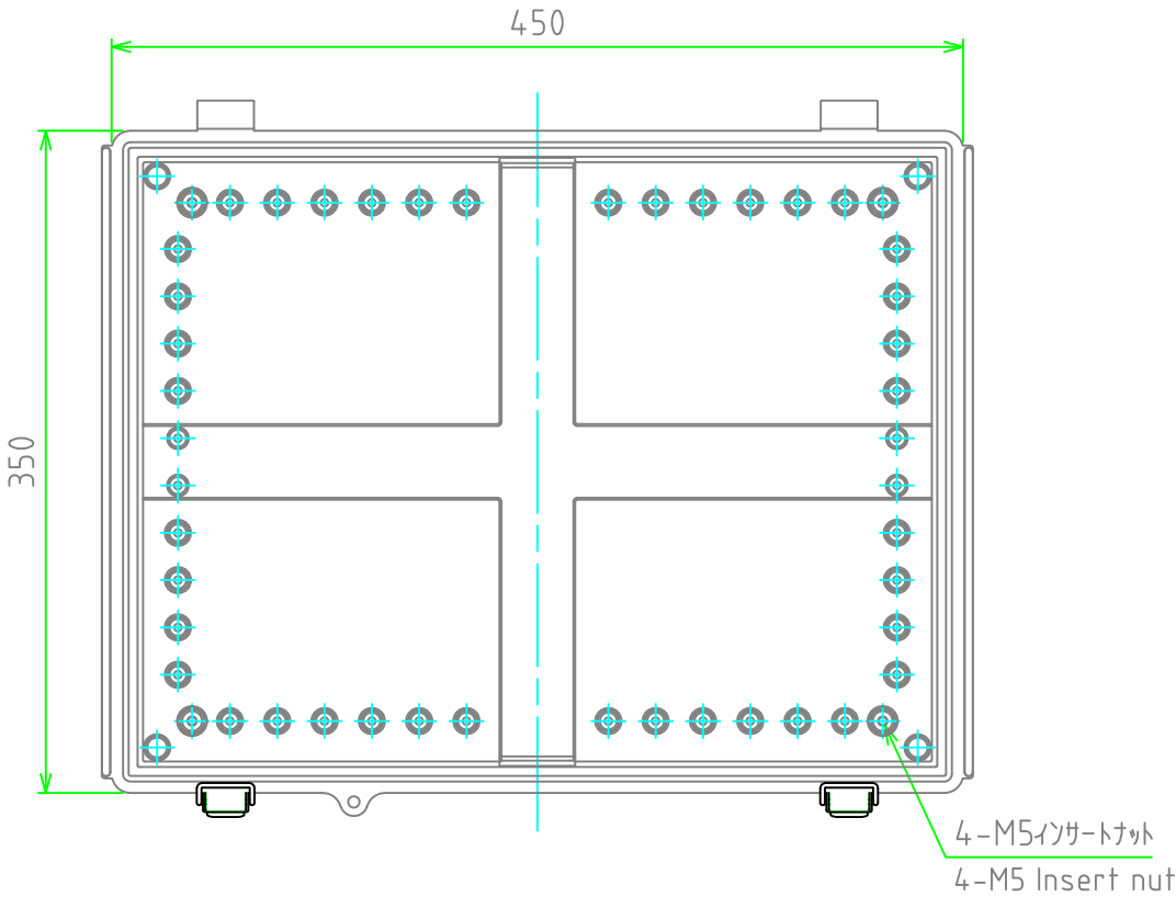
ボディー(内視) Base (Internal View)
