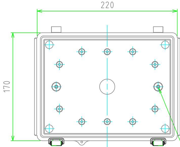
ボディー(内視) Base (Internal View)
