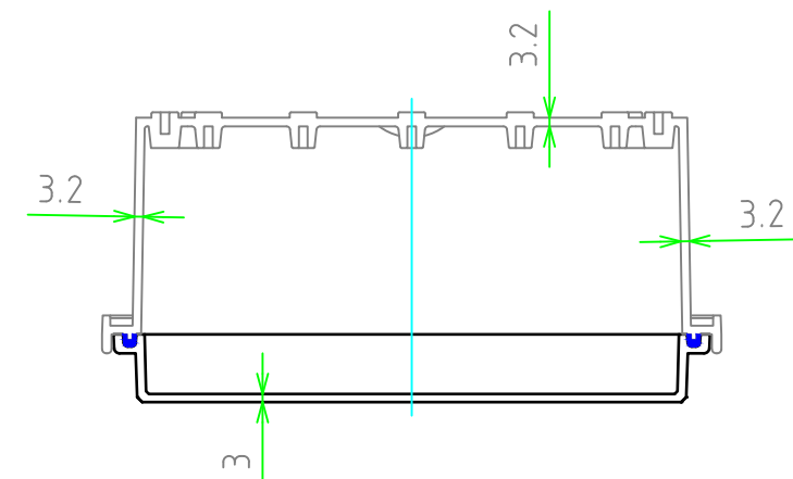
ボディー (内視) Base (Internal View)
