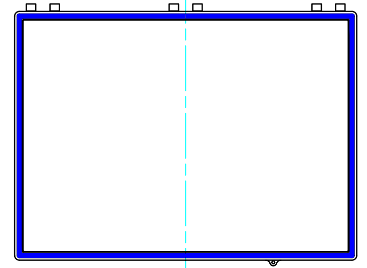
6-M5インサートナット 6-M5 Insert nut
