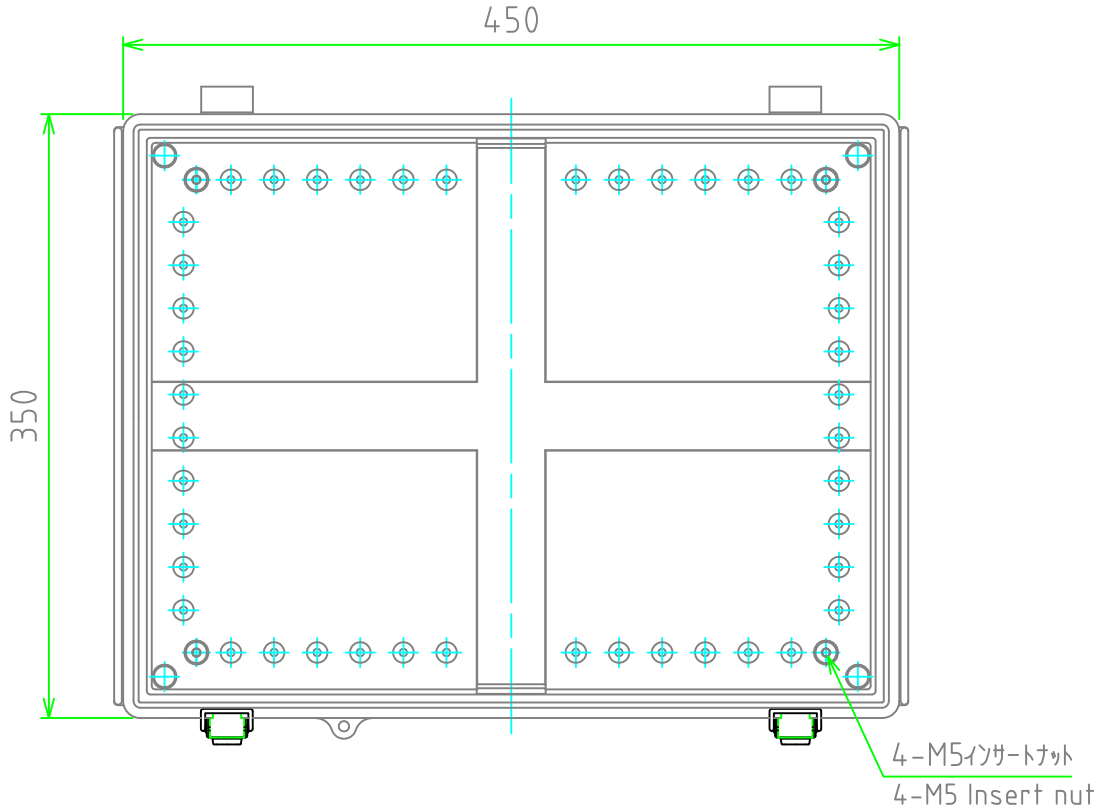
ボディー(内視) Base (Internal View)
