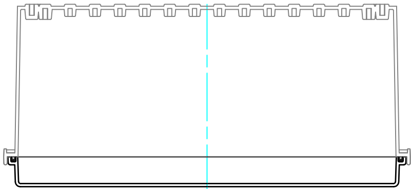
ボディー(内視) Base (Internal View)
