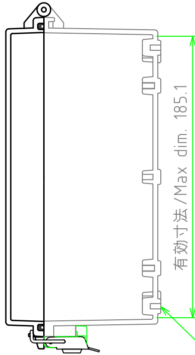
4-M4インサートナット 4-M4 Insert nut
