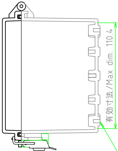
2-M4インサートナット 2-M4 Insert nut
