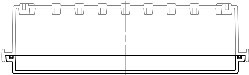
ボディー(内視) Base (Internal View)
