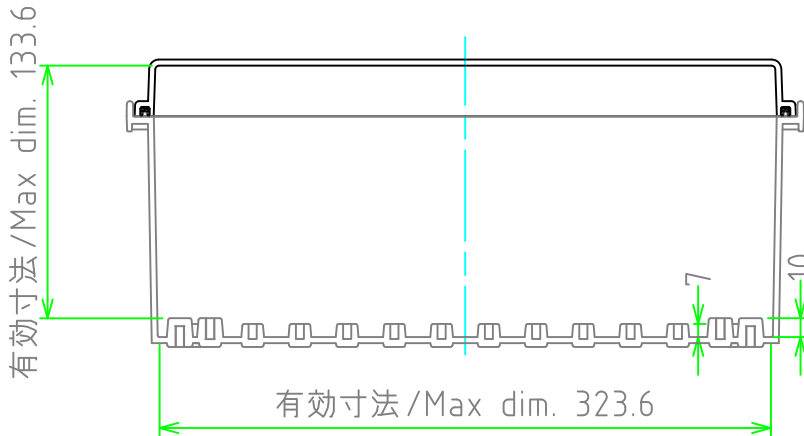
4-M5インサートナット 4-M5 Insert nut
