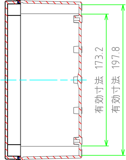
D-D
